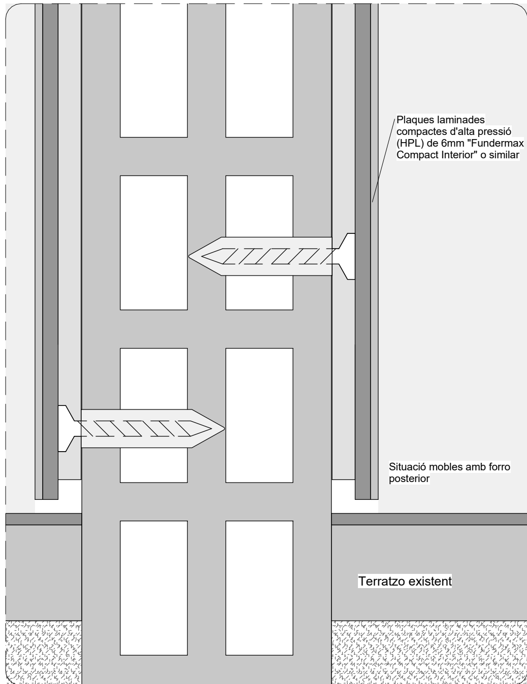
DET-HAB-TAU+EST (ido) (e 1 : 1)
