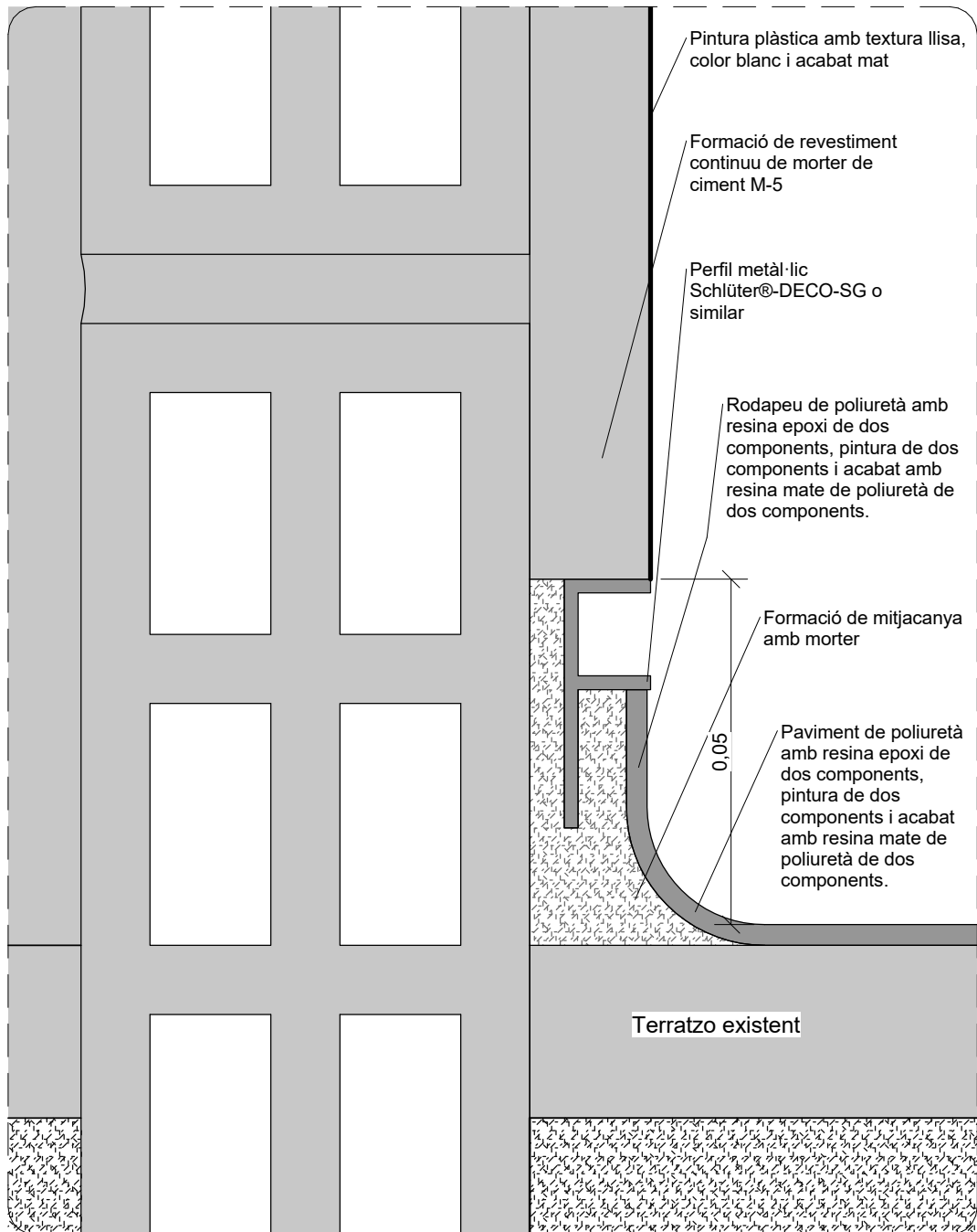
B3-DET3 (e 1 : 1)
